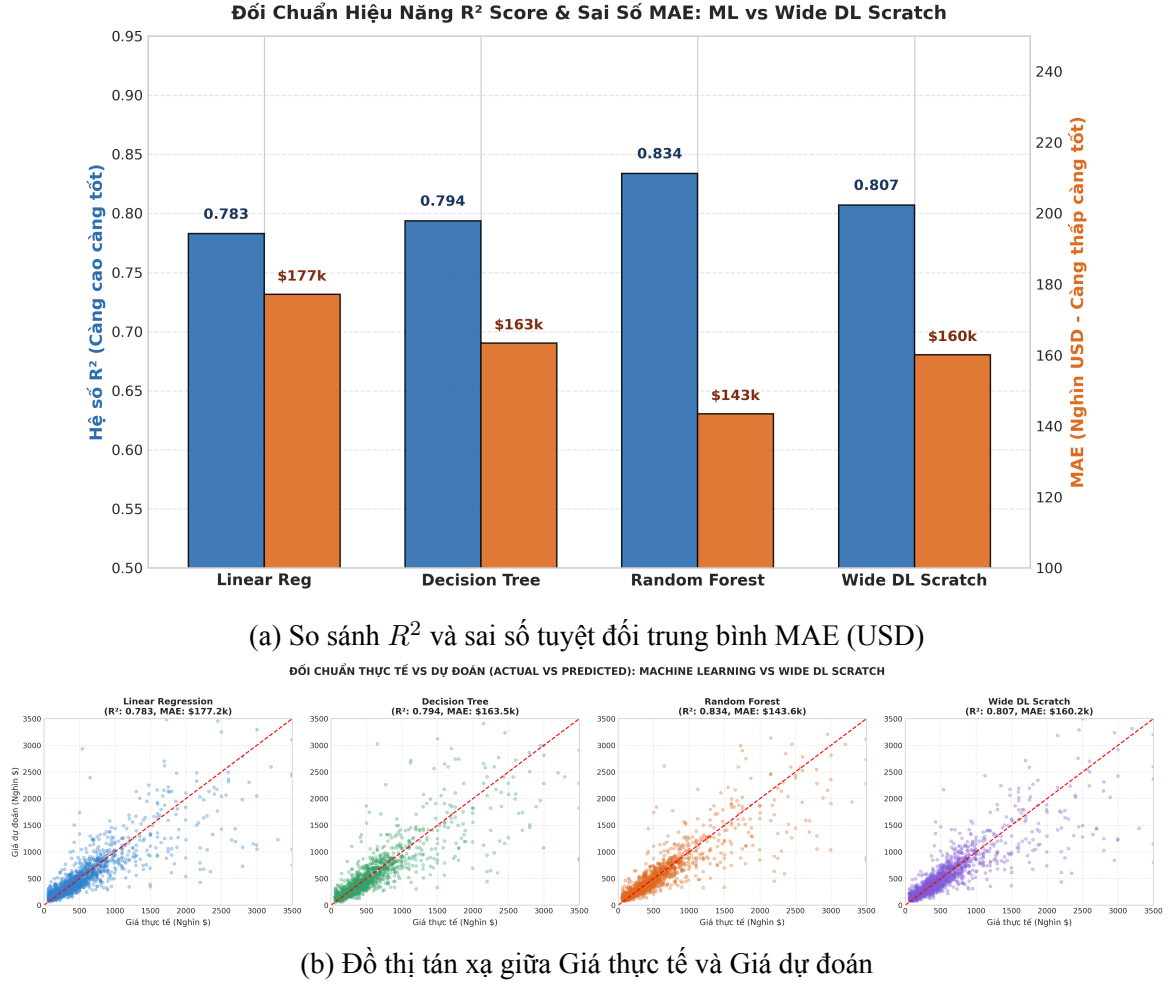
Figure 4.5: Đối chuẩn trực quan hiệu năng hệ thống định giá bất động sản
