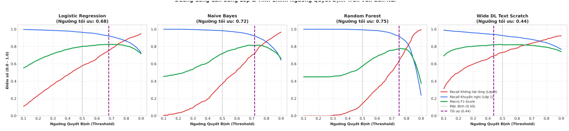
Figure 5.4: Đường cong cân bằng lớp và tính chỉnh ngưỡng quyết định trên văn bản NLP
