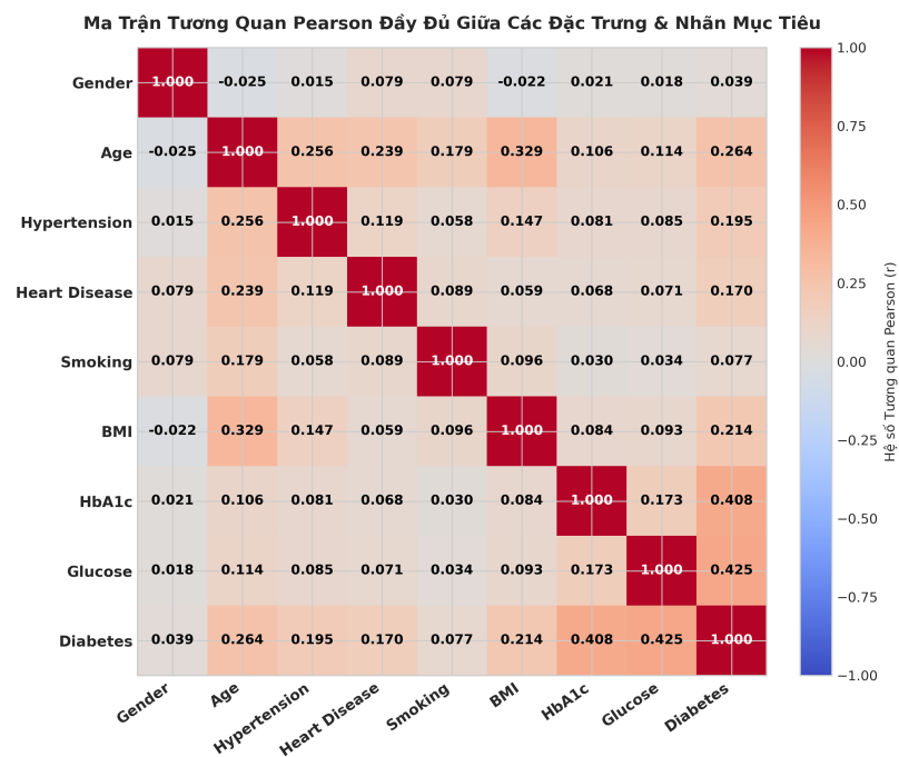
(b) Ma trận tương quan Pearson giữa các đặc trưng
